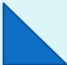
ορθογώνιο τρίγωνο
