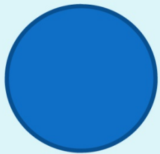
κύκλος
