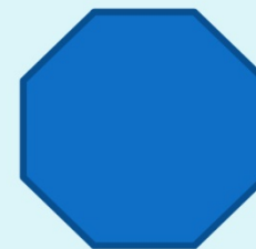
οκτάγωνο
