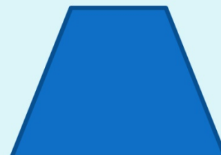
τραπέζιο
